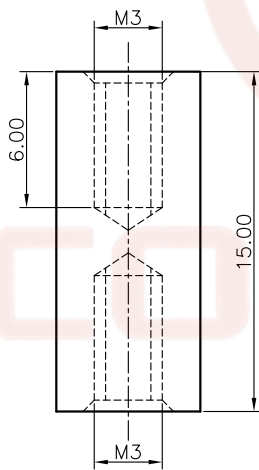
5.5x15mm M3 Nut
